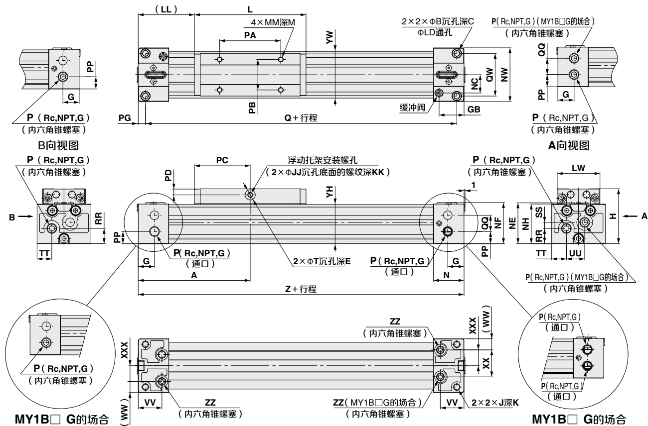
标准配管/集中配管共通
