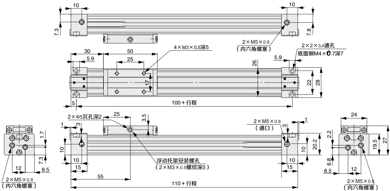
外形尺寸图
