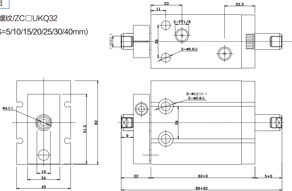
外形尺寸图
